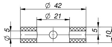
Przekrój Y-Y
