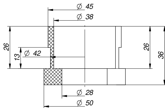
Przekrój Z-Z
