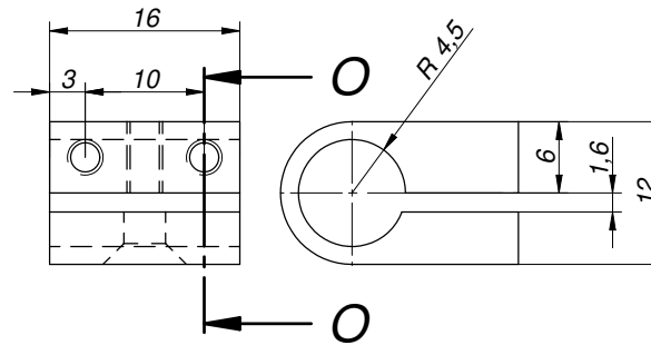
Przekrój O-O
