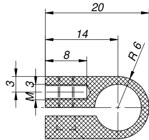
Przekrój O-O
