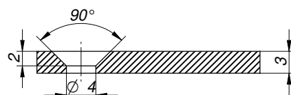
Przekrój L-L
