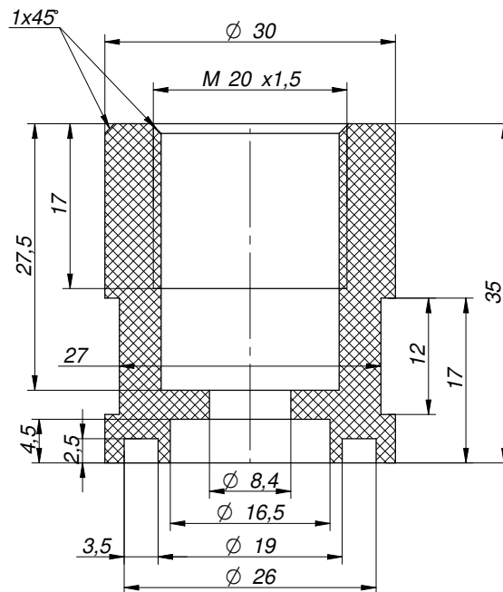
Przekrój AB-AB
