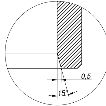
Szczegół U
