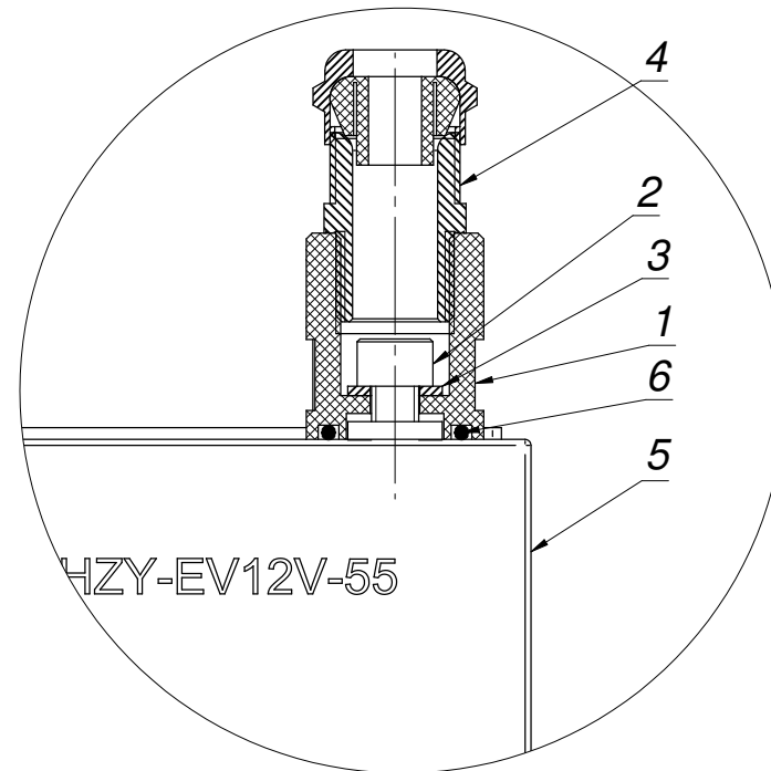
Szczegół D
