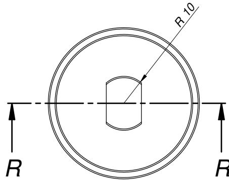
Szczegół U
