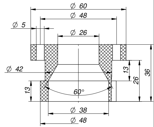
Przekrój X-X
