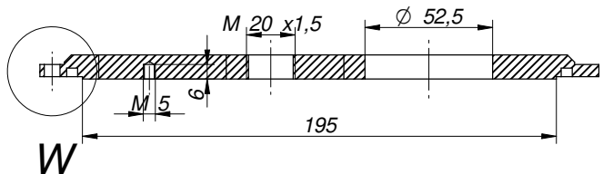
Przekrój V-V
