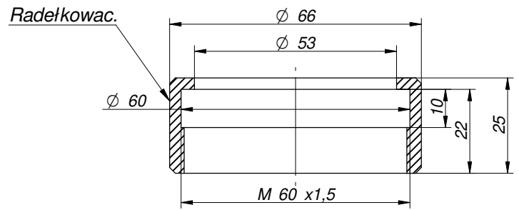
Przekrój S-S
