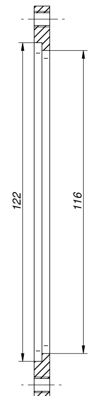
Przekrój H-H
