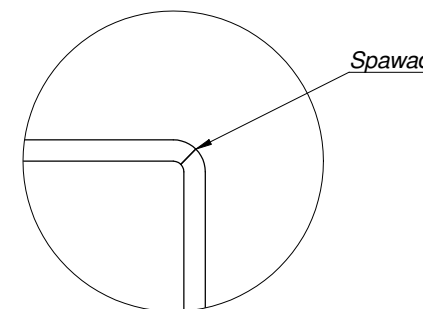
Szczegół I
