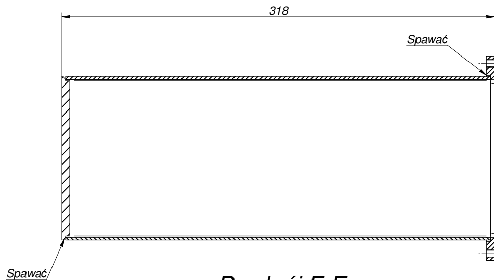
Przekrój E-E
