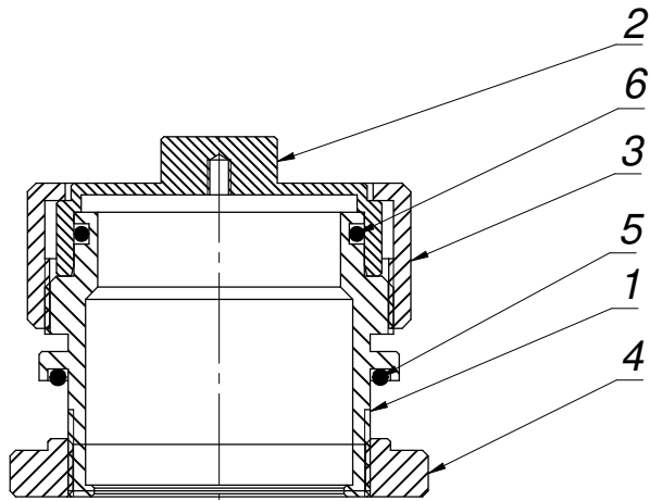
Przekrój F-F
