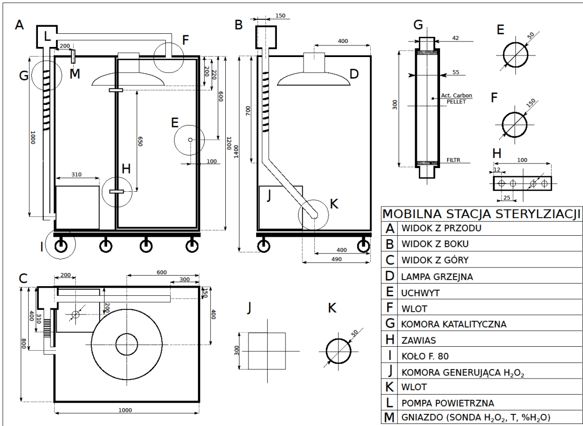
Rys. 1. Roboczy schemat konstrukcji prototypu mobilnej stacji sterylizacji.
