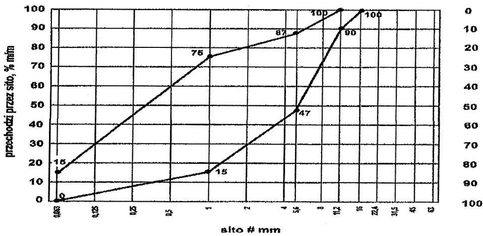
Rys. 2. Krzywe graniczne uziarnienia mieszanki kruszywa niezwiązanego 0/11,2 mm do nawierzchni
