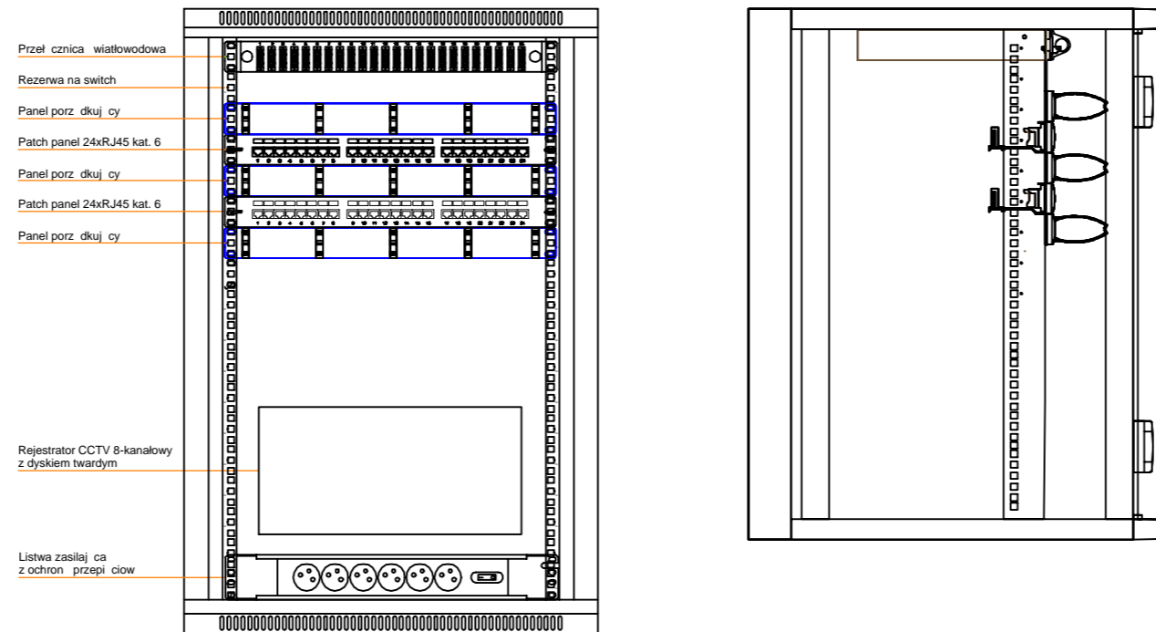
WIDOK ELEWACJI SZAFKI LPD-1/D Szafa na cienna dzielona 19" 18U Wymiary 910x600x600
