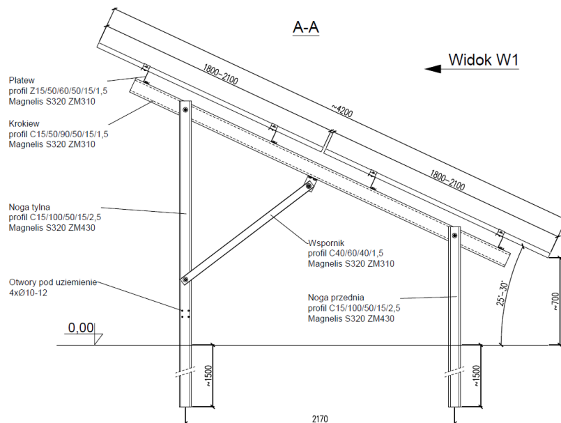
Rys.4. Przykładowa konstrukcja montażowa rzędowa. Systemy-wolnostojace/system-wbijany-dwupodporowy-2-moduly-w-pionie/ kierunek południe
