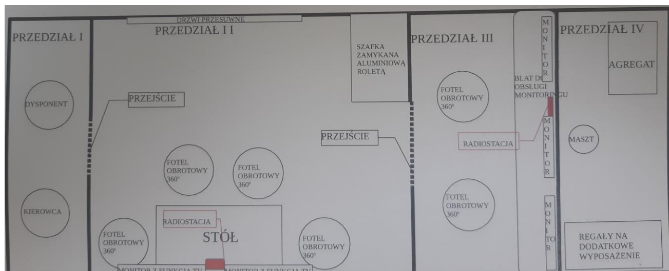
Rysunek 1: Rzut z góry, pojazd MCWTiD
