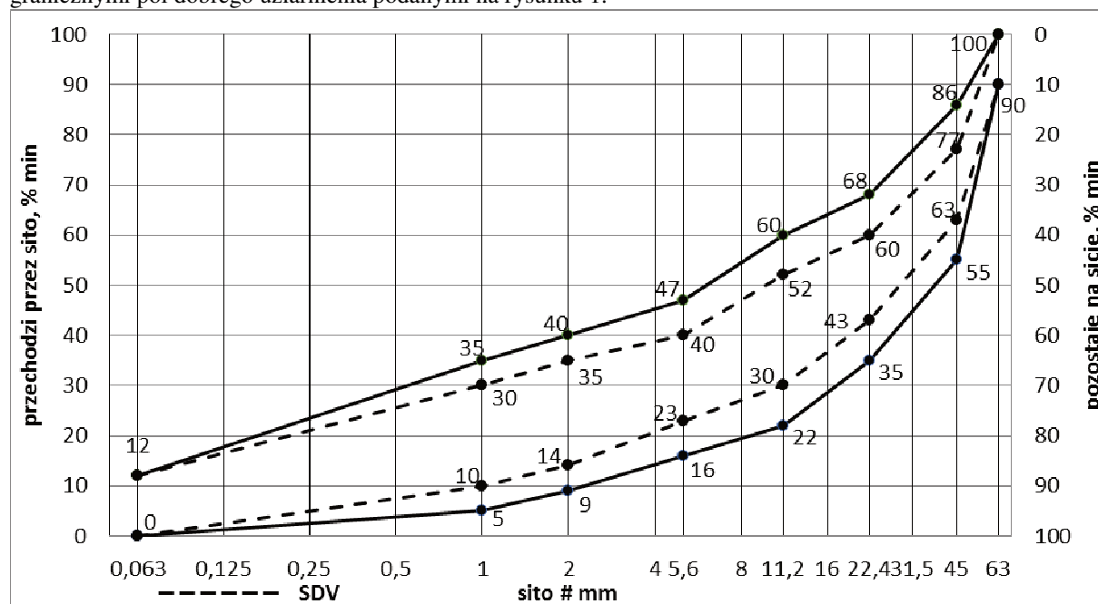
Rysunek 1. Mieszanka niezwiązana 0/63 do warstwy ulepszanego podłoża stabilizowanego georusztem
