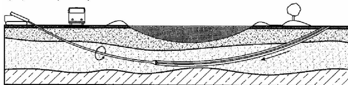
Rys.2) Poszerzanie otworu
