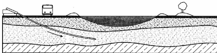
Rys.1) Przewiert pilotażowy
