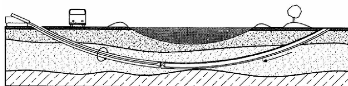
Rys.3) Przeciąganie rurociągu
