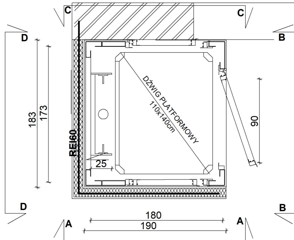
Rzut na kondygnacji 3 i 4 1:25
