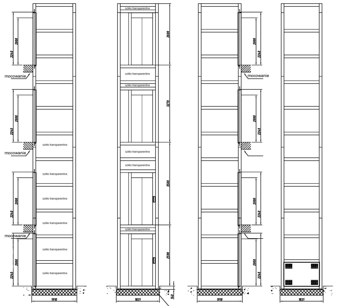
Widok A-A 1:100 Widok B-B 1:100 Widok C-C 1:100 Widok D-D 1:100
