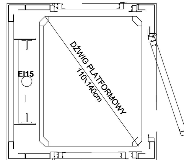
SZKLANE PANELE W ŚCIANCE DŹWIGU
