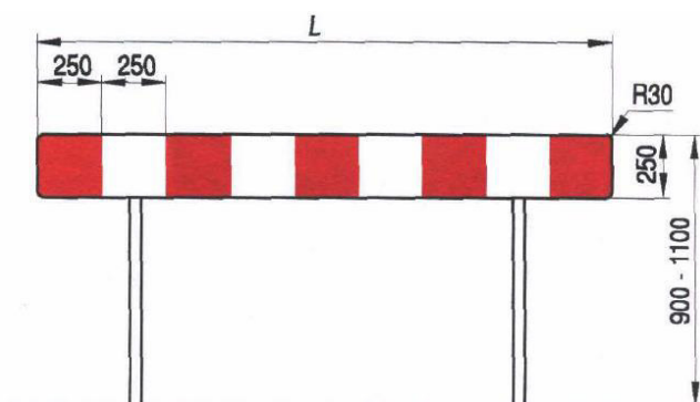
Rys. 1. Zapora drogową pojedynczą U-20a
