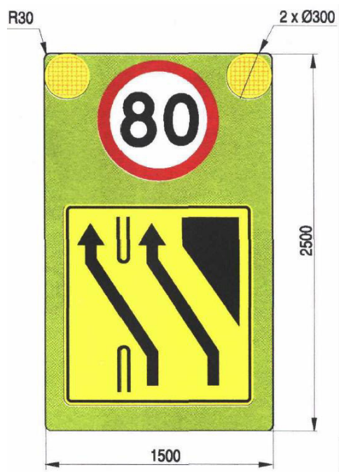
Rys. 21. Tablica wczesnie ostrzegajaca U-27
