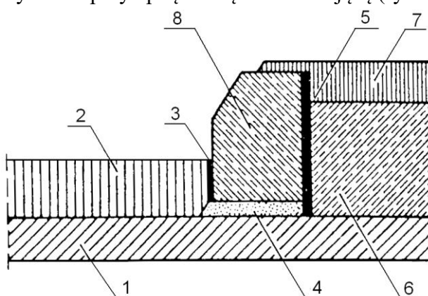
Rys. 4.1. Przykład wykonania krawężnika: 1 - warstwa wiążąca, 2 - warstwa ścieralna, 3 - samoprzylepna taśma uszczelniająca połączenie warstwy ścieralnej z krawężnikiem, 4 - łoża pod krawężnik z mieszanki mineralno-asfaltowej, 5 - masa zalewowa w złączeniu podłużnym, 6 - płyta betonowa, 7 - warstwa ścieralna z asfaltu lanego na chodniku, 8 - krawężnik kamienny
