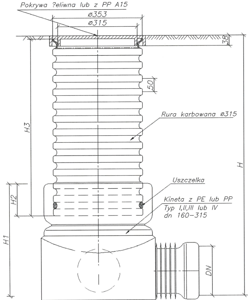
Studzienka inspekcyjna \varnothing 315 z pokryw? ?eliwn? lub z PP klasy A15
