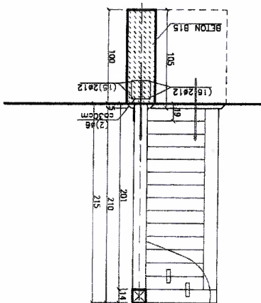
PRZEKRÓJ 3-3
