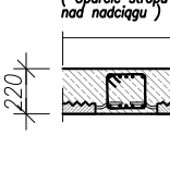
Det. 03 skala 1:40 (Oparcie stropu nad nadciągiem)
