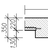
Det. 05 skala 1:40
