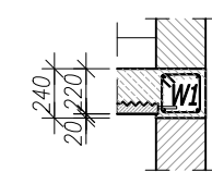
Det. 02 skala 1:40
