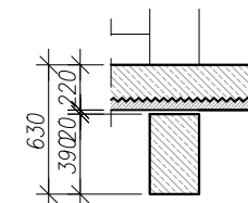
Det. 01 skala 1:40
