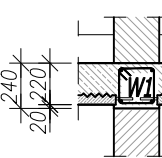
Det. 04 skala 1:40
