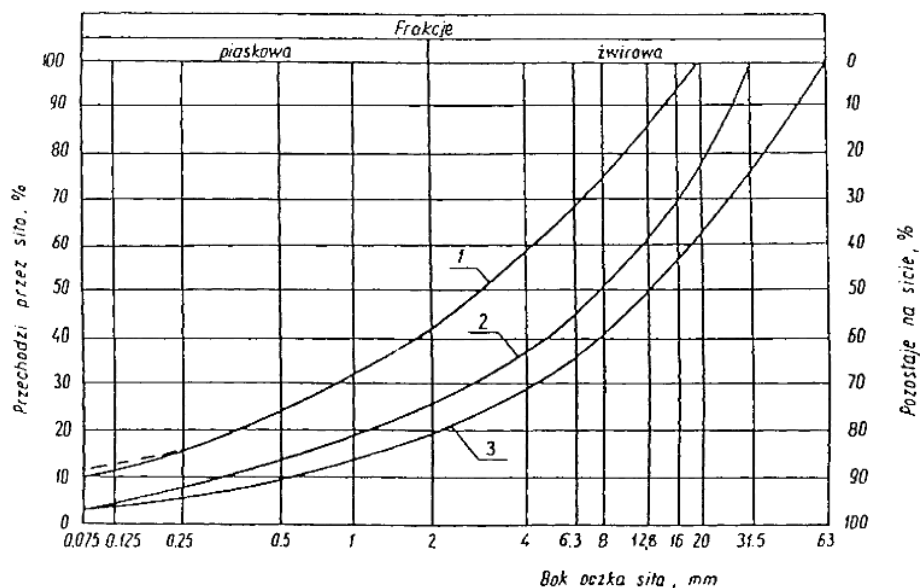
Rysunek 1. dobrego uziarnienia kruszyw
