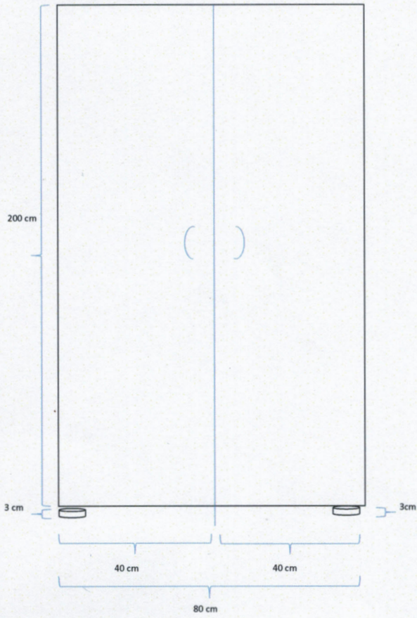
Szafa na ubrania – widok z przodu
