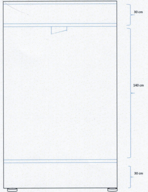
Szafa na ubrania – widok z przodu bez drzwi z wieszakiem na ubrania
