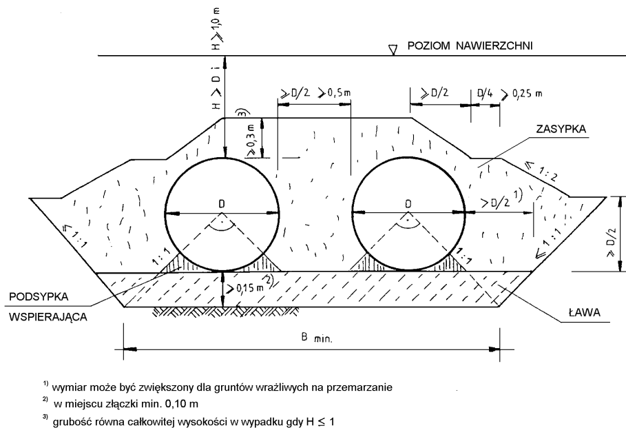
Rys. 9. Zasyпка nad przepustem dwururowym
