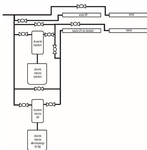
Ryc. 1. Schemat modyfikacji rur rozprzewadzających wodę i nawóz
