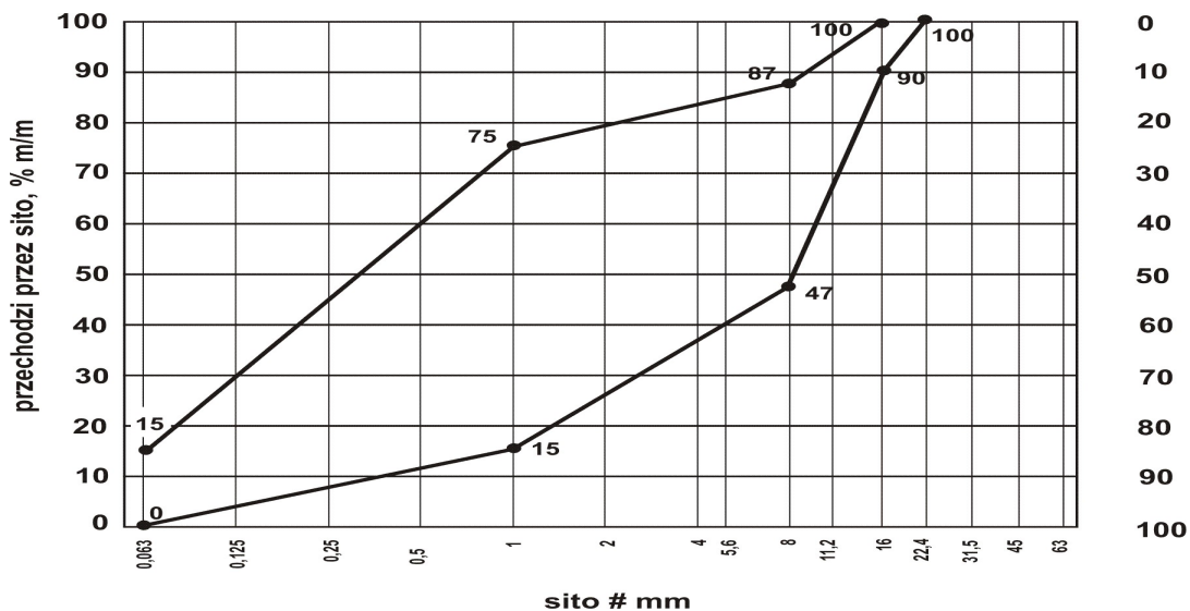
Rys. 3. Uziarnienie mieszanki niezwiązanej 0/16 dla warstwy mroзоochronnej
