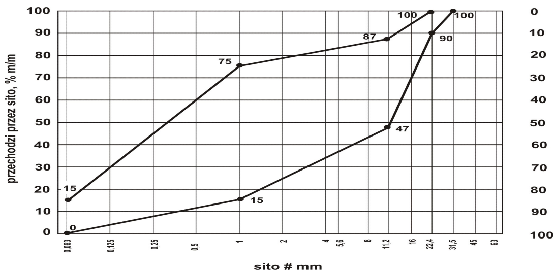
Rys. 4. Uziarnienie mieszanki niezwiązanej 0/22, 4 dla warstwy mroзоochronnej
