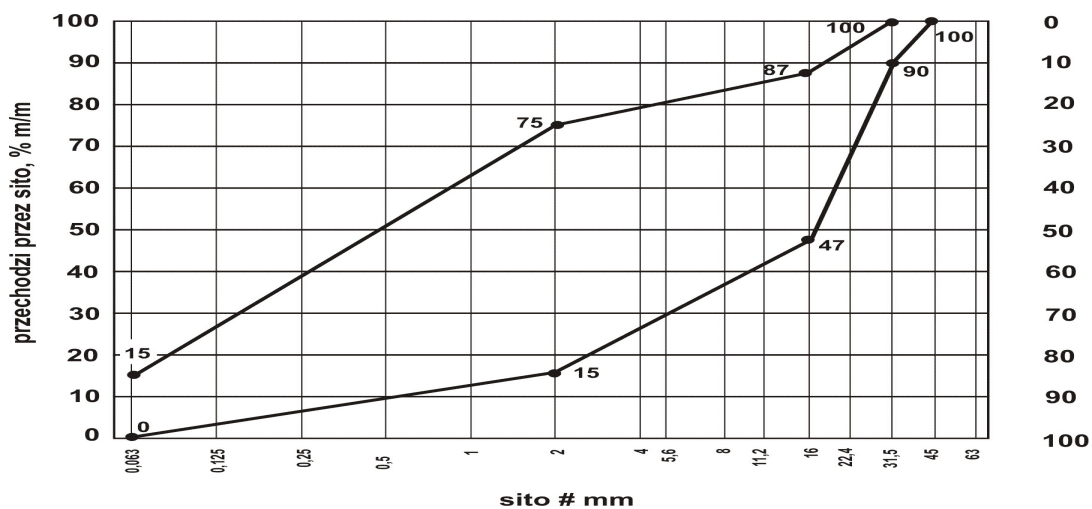
Rys. 5. Uziarnienie mieszanki niezwiązanej 0/31,5 dla warstwy mroзоochronnej
