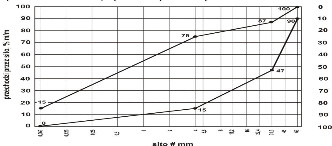
Rys. 7. Uziarnienie mieszanki niezwiązanej 0/63 dla warstwy mrozoochronnej
