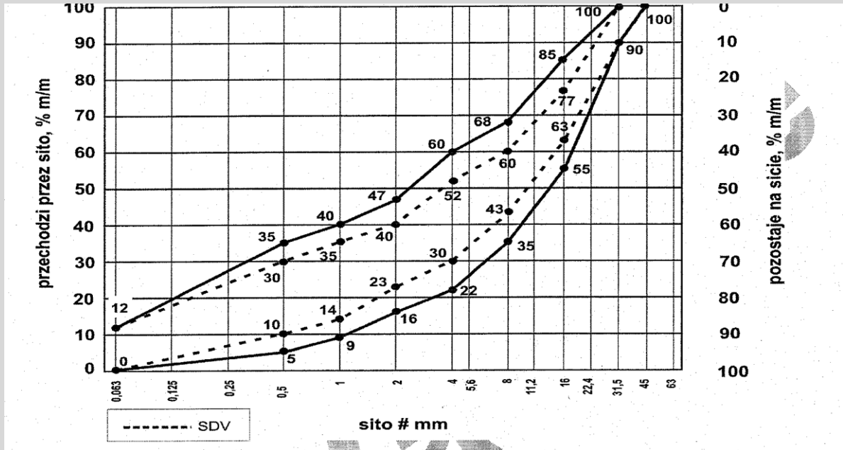
Rys. 1. Mieszanka niezwiązana 0/31,5 do warstwy podbudowy pomocniczej
