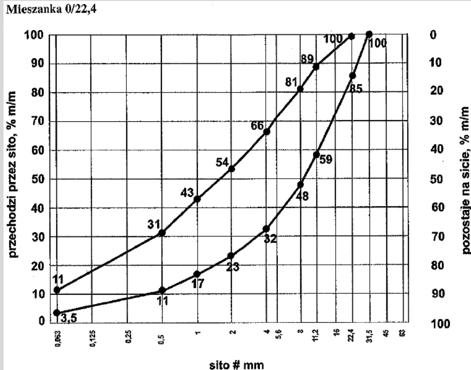
Rys. 1. Uziarnienie mieszanki CBGM 0/22,4
