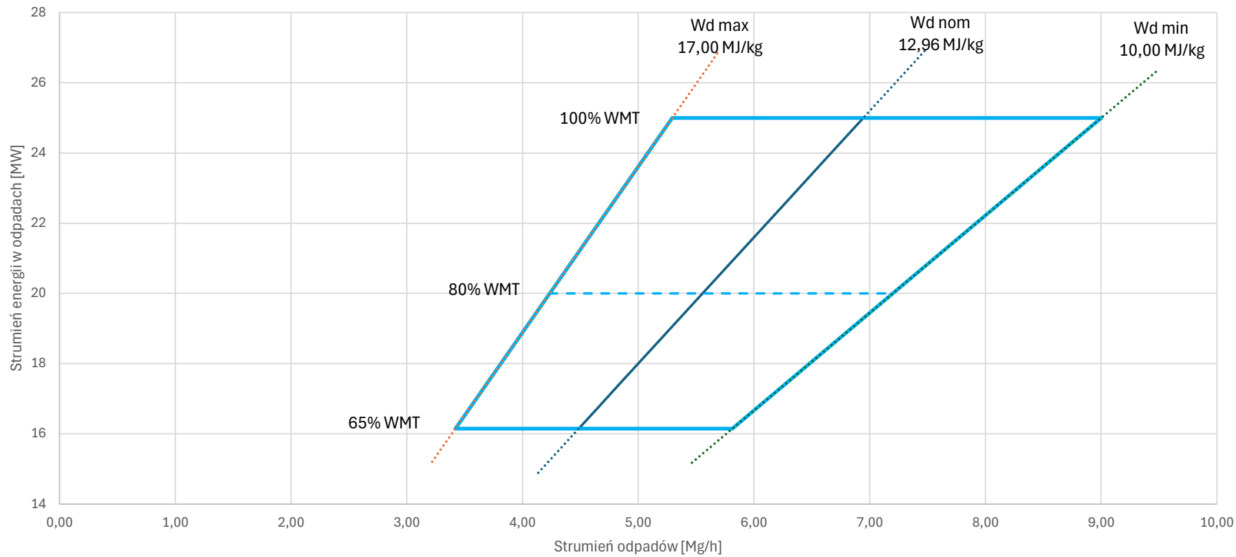
Wykres spalania
