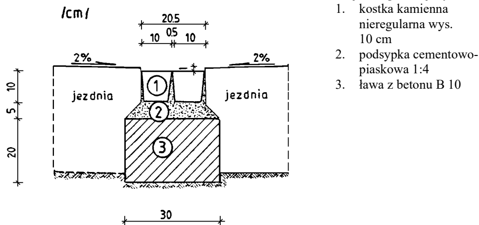
Rys. 2.2. Ściek międzyjezdniowy z dwóch rzędów kostki kamiennej nieregularnej wysokości 10 cm
