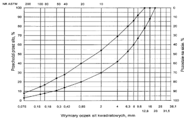
Rys. 5. Krzywe graniczne uziarnienia mieszanki mineralnej BA od 0 do 12,8 mm do warstwy wiążącej, wyrównawczej i wzmacniającej nawierzchni drogi o obciążeniu mchem KR1 lub KR2
