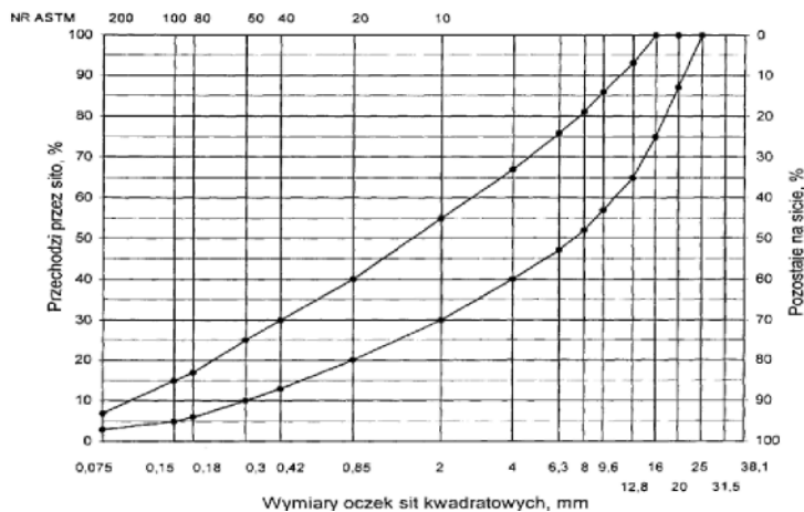
Rys. 4. Krzywe graniczne uziarnienia mieszanki mineralnej BA od 0 do 16 mm do warstwy wiążącej, wyrównawczej i wzmacniającej nawierzchni drogi o obciążeniu mchem KR1 lub KR2
