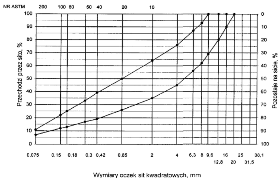
Rys. 2. Krzywe graniczne uziarnienia mieszanki mineralnej BA od 0 do 8 mm, od 0 do 6,3 mm do warstwy ścieralnej nawierzchni drogi o obciążeniu mchem nawierzchni drogi o obciążeniu ruchem KR1 lub KR2
