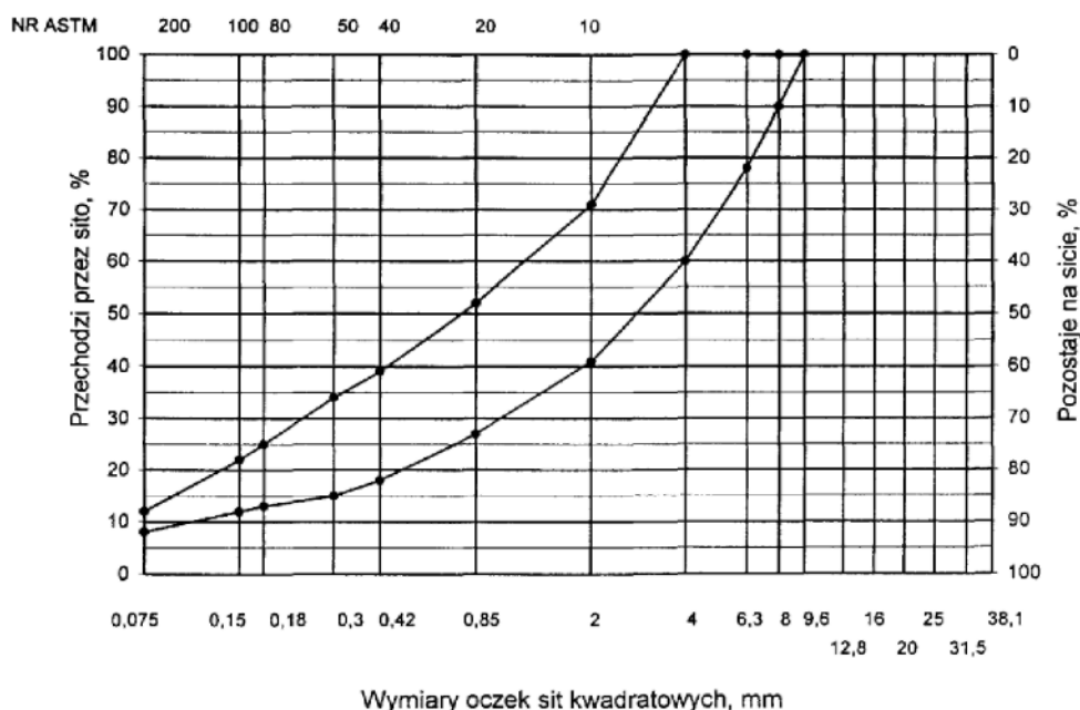
Rys. 2. Krzywe graniczne uziarnienia mieszanki mineralnej BA od 0 do 8 mm, od 0 do 6,3 mm do warstwy ścieralnej nawierzchni drogi o obciążeniu mchem nawierzchni drogi o obciążeniu ruchem KR1 lub KR2
