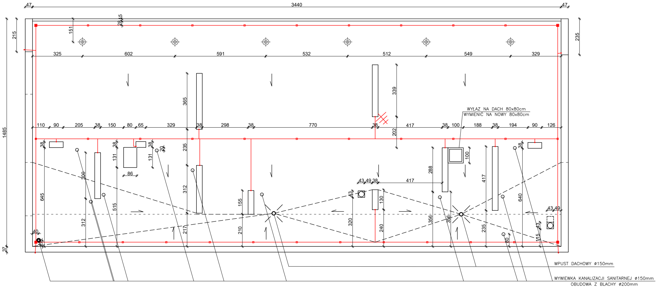
RZUT DACHU
