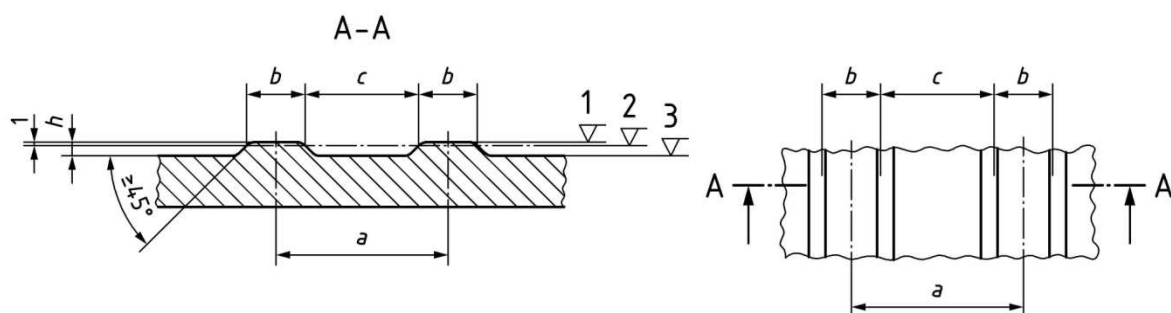
Rys. 1a. Płytki kierunkowa przewodząca- szczegóły powierzchni
