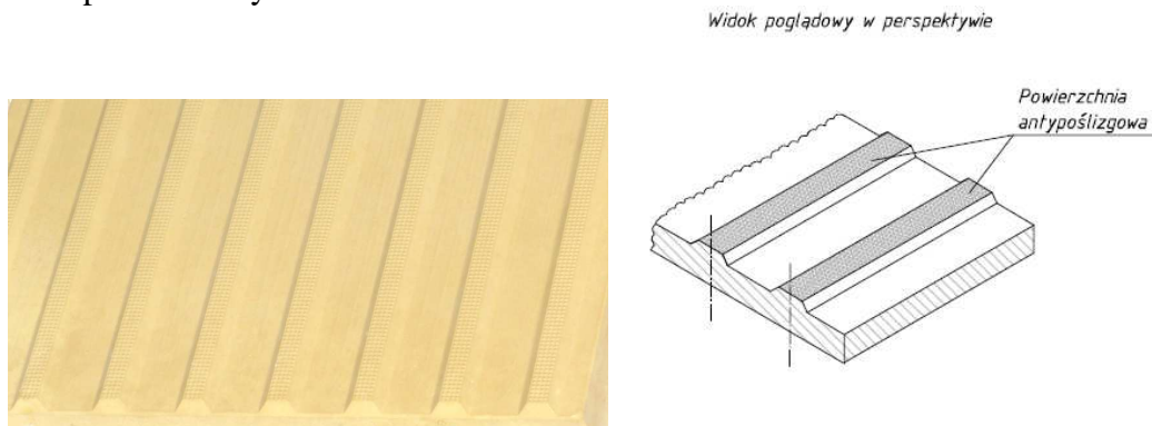
Rys. 1a. Płytki kierunkowa przewodząca- szczegóły powierzchni
