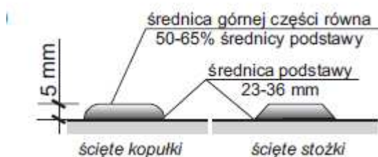
Rys. 2a. Płytki ostrzegawcza – szczegóły powierzchni
