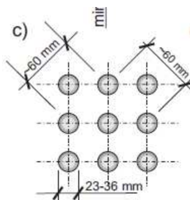
Rys 1b. Wymiary wypustek płytki przewodzącej na podstawie normy DIN 32984
