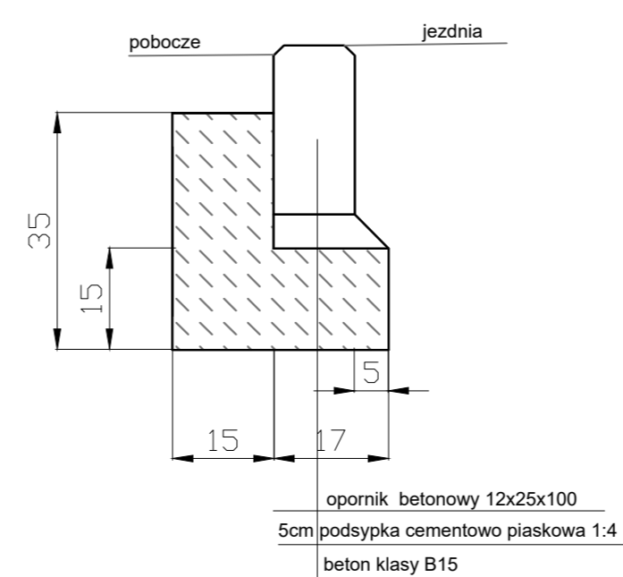
opornik betonowy 12x25 cm
