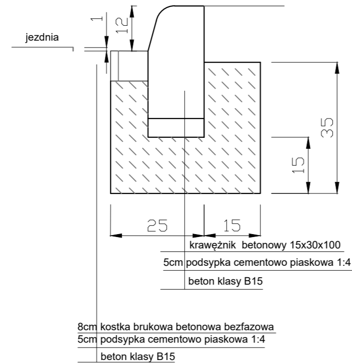
krawężnik betonowy 15x30 cm na ławie betonowej ściek betonowy szer 10cm na ławie betonowej
