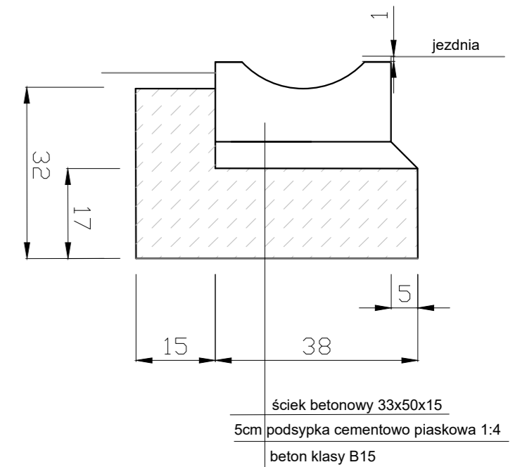
ściek betonowy szer 33cm na ławie betonowej
