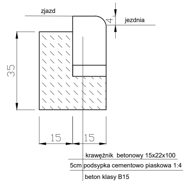
krawężnik betonowy - zjazd 15x22 cm
