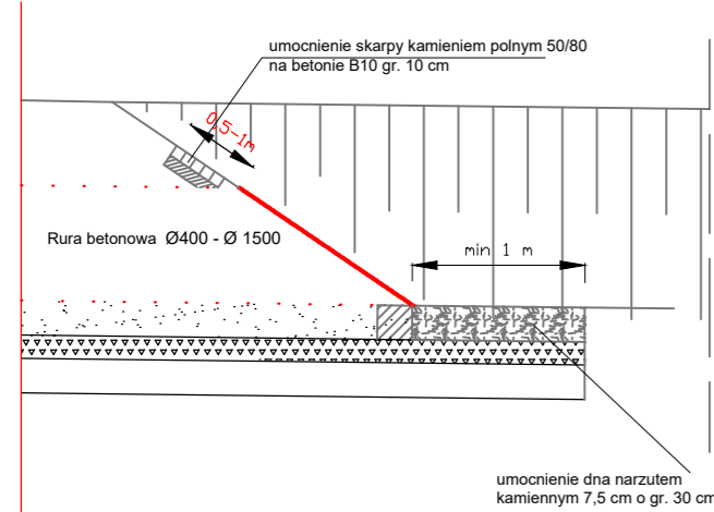
Umocnienie skarpy - wylot przepustu
