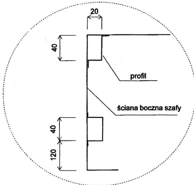
Szczegół B
