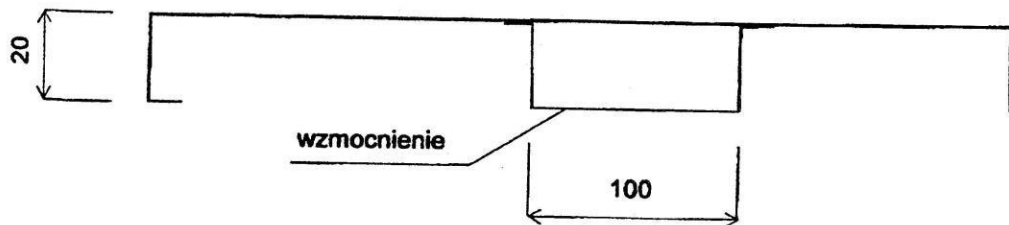
Półka przestawna
