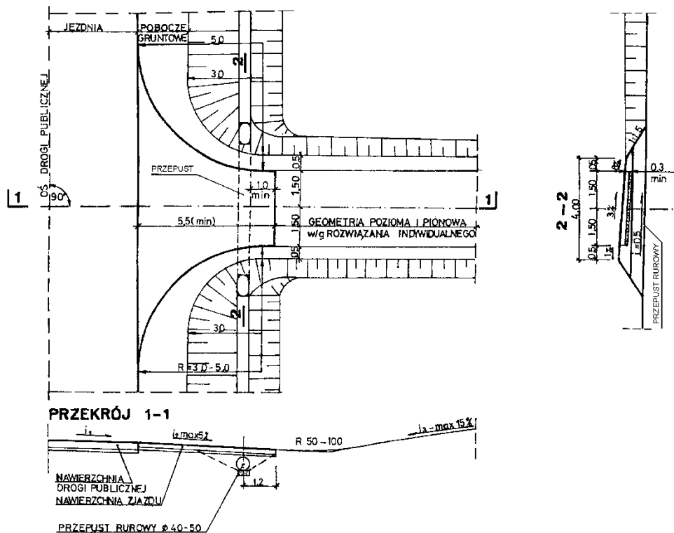
Rys. 3.1. Przykładowe rozwiązanie sytuacji zjazdu indywidualnego z przepustem
