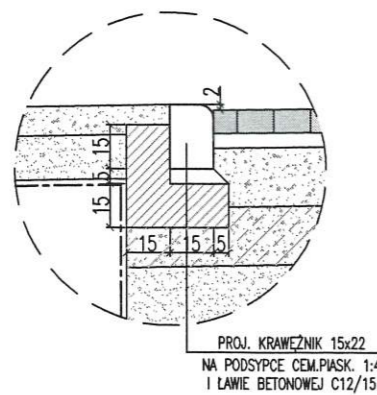
SZCZEGÓŁ KONSTRUKCYJNY A1 KRAWĘŻNIKA NAJAZDOWEGO 1:25
