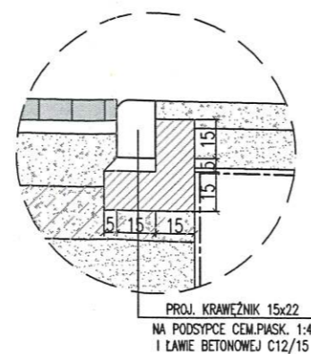
SZCZEGÓŁ KONSTRUKCYJNY A2 KRAWĘŻNIKA NAJAZDOWEGO 1:25
