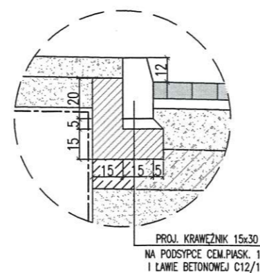
SZCZEGÓŁ KONSTRUKCYJNY B KRAWĘŻNIKA WYSTAJĄCEGO 1:25
