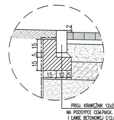
SZCZEGÓŁ KONSTRUKCYJNY C OPORNIKA 1:25
