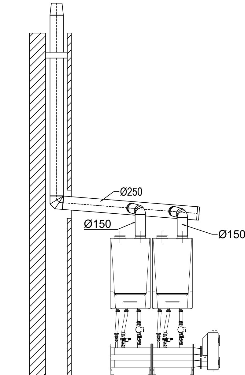
System kominowy kaskadowy ze stali kwasoodpornej
