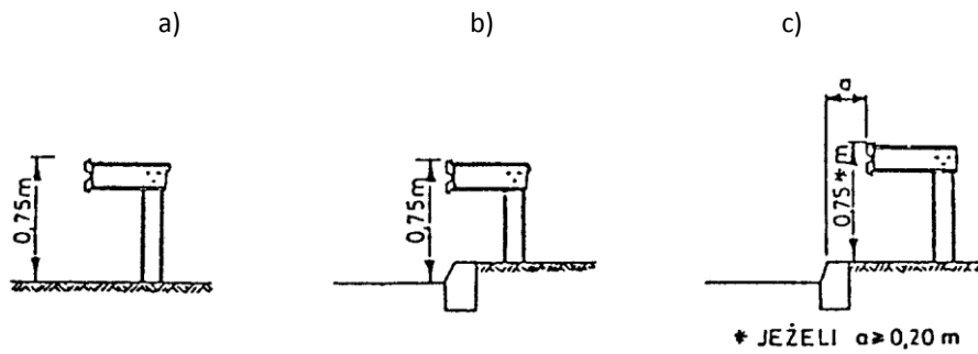
Załącznik 11.4. Profilowana taśma stalowa typu A i B, wg L. Mikołajków: Drogowe bariery ochronne, WKiŁ, 1983
