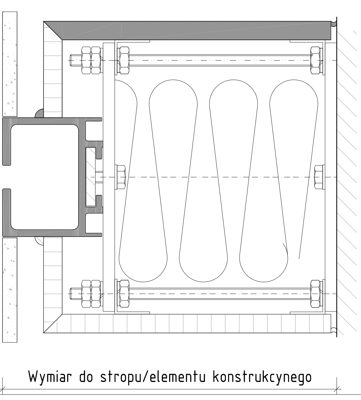
Szyba aluminiowa – zawieszenie podwójne
