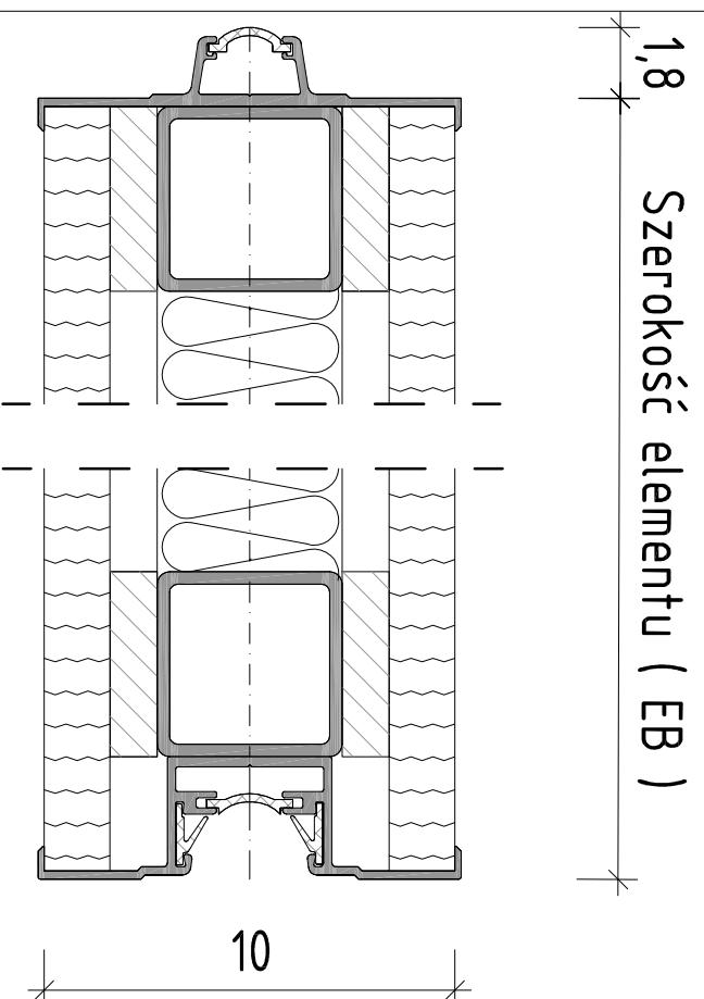
Rama stalowa Profile aluminiowe z listwą magnetyczną
