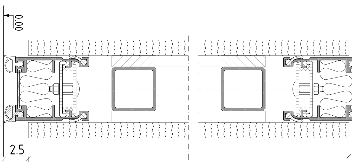
Rama stalowa Profile aluminiowe z listwą magnetyczną
