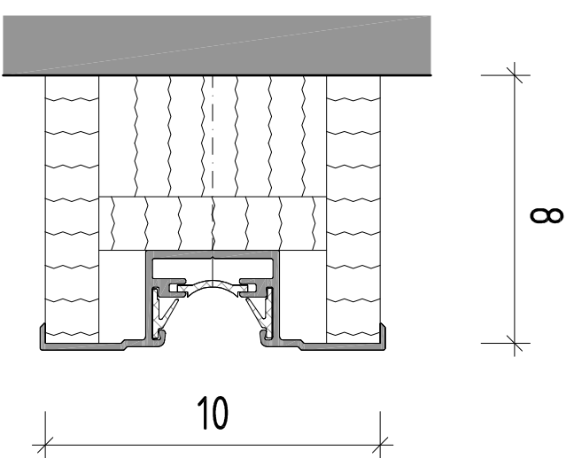
Profil przysięcienny Profil aluminiowy z listwą magnetyczną
