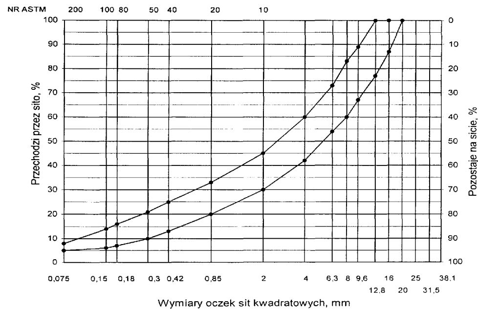
13. Krzywe graniczne uziarnienia mieszanki mineralnej BA od 0 do 16 mm do warstwy wyrównawczej nawierzchni drogi o obciążeniu ruchem od KR3 do KR6
