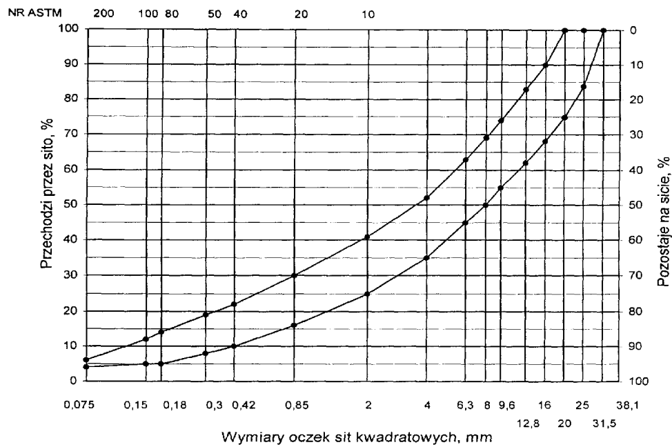
11. Krzywe graniczne uziarnienia mieszanki mineralnej BA od 0 do 25 mm do warstwy wiążącej, wyrównawczej i wzmacniającej nawierzchni drogi o obciążeniu ruchem od KR3 do KR6
