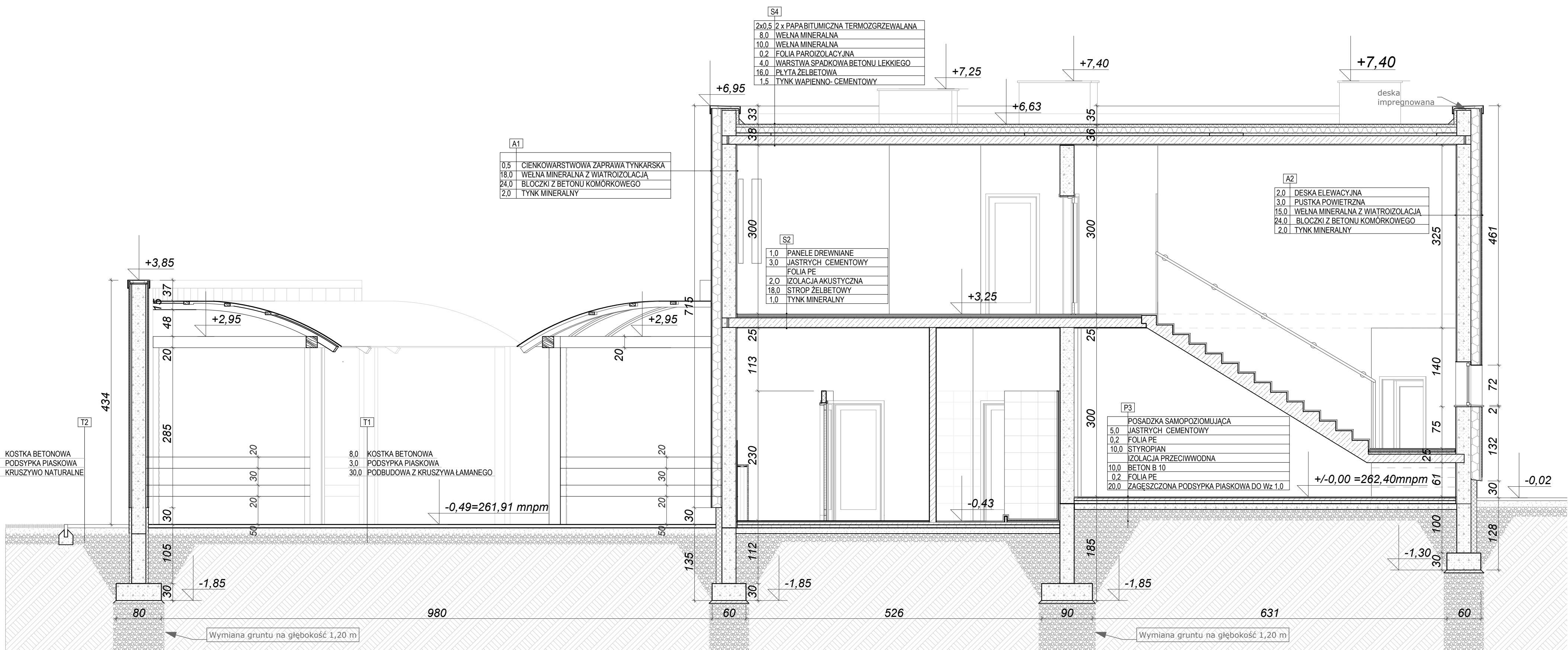
PRZEKRÓJ A-A SKALA 1:50
