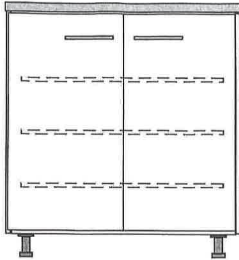
szafka 85x80x60 poz. 25
