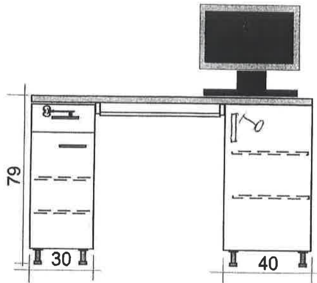
poz. 50 biurko komputerowe z szafką 79x132x70
