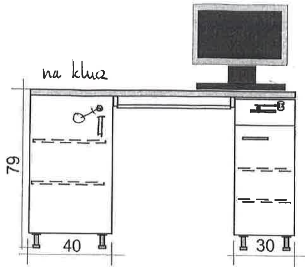
biurko komputerowe z szafką 79x132x70 poz. 13
