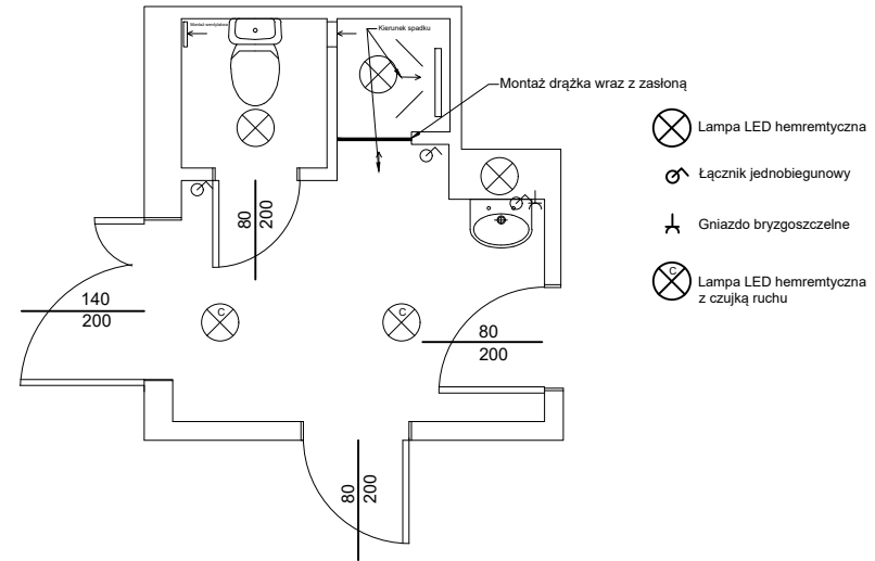
Łazienka budynek B piwnica - stan projektowany
