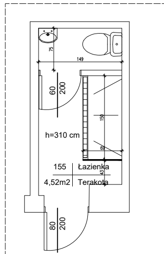
Łazienka budynek B piętro - stan istniejący
