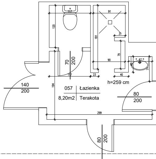
Łazienka budynek B piwnica - stan istniejący
