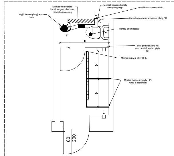
Łazienka budynek B piętro - stan projektowany
