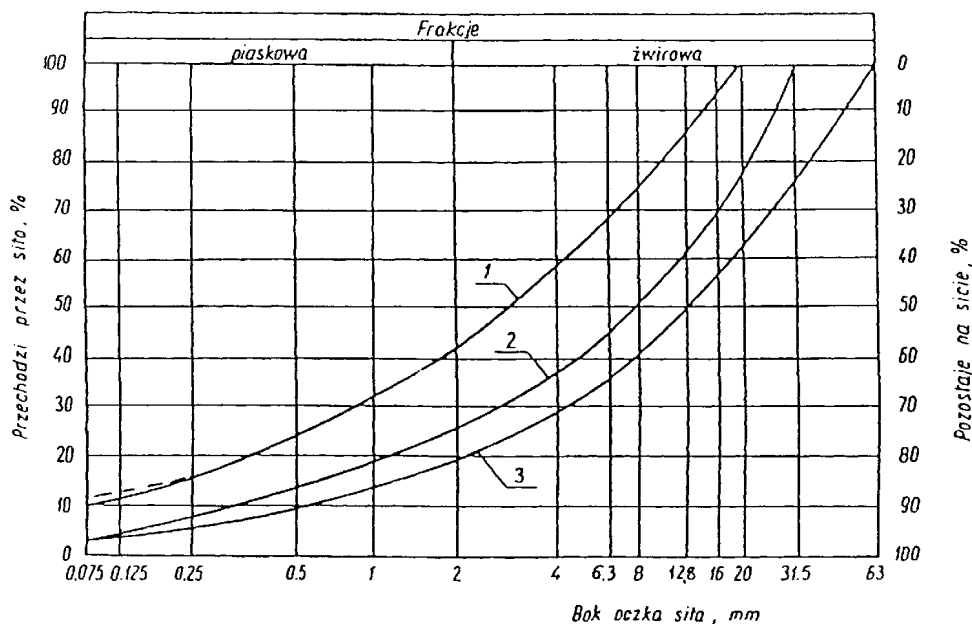
Rysunek 1. Pole dobrego uziarnienia kruszyw przeznaczonych na podbudowy wykonywane metodą stabilizacji mechanicznej. 1-2 kruszywo na podbudowę zasadniczą (górną warstwę) lub nawierzchnię 1-3 kruszywo na podbudowę pomocniczą (dolną warstwę).
