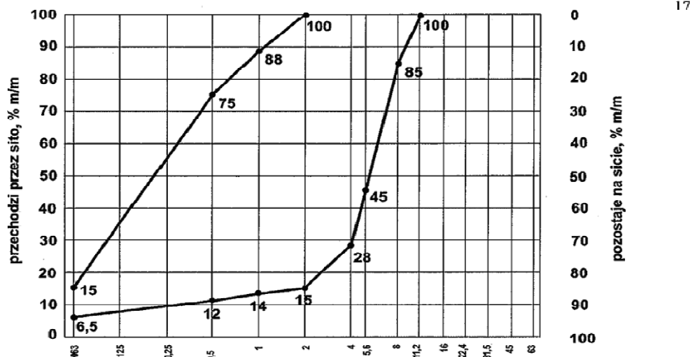
Rys. 5.5. Uziarnienie mieszanki CBGM 0/8
