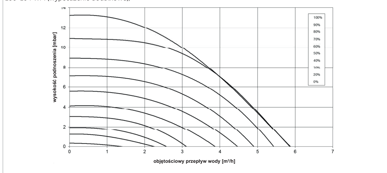
Rysunek 8. Wysokość podnoszenia pompy w kotle WGB 50 i (pompa obiegowa c.o. o wysokiej sprawności typ HEP 25-180-10 PWM [wyposażenie dodatkowe])
