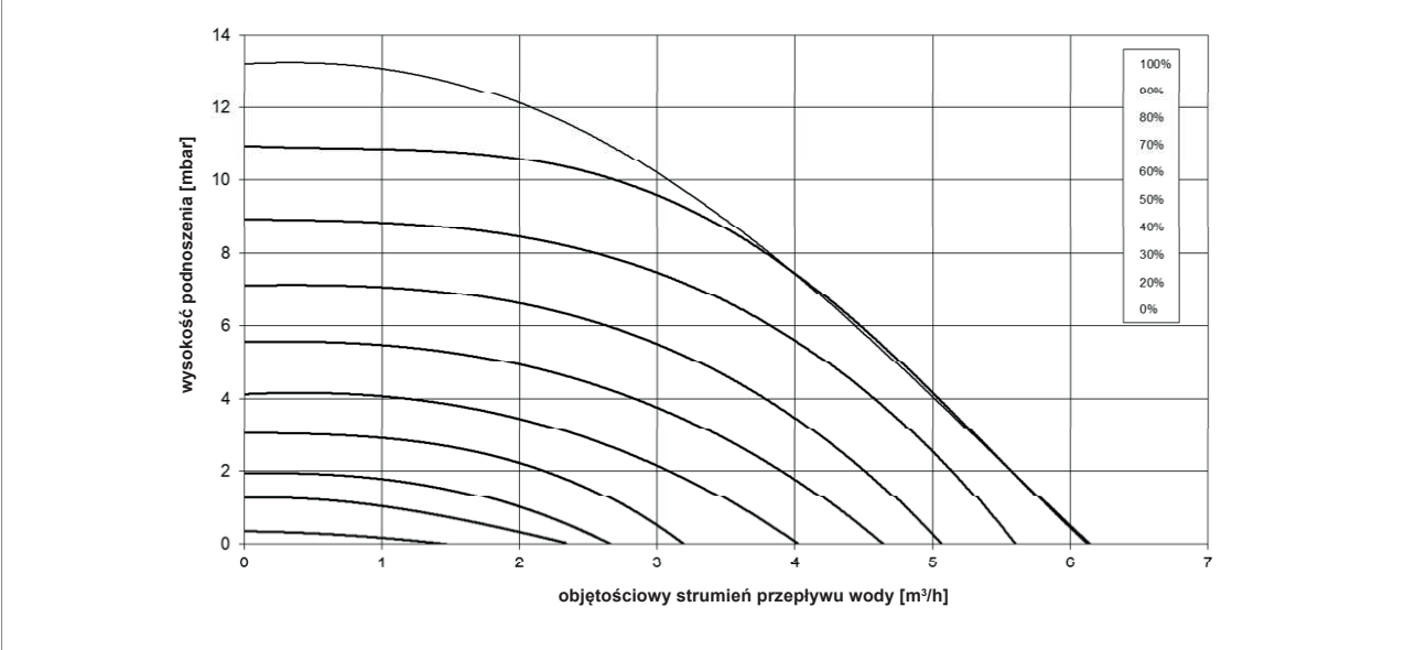
Rysunek 9. Wysokość podnoszenia - pompy w kotle WGB 70-110 i (pompa obiegowa o wysokiej sprawności typ HEP 25-180-10 PWM [wyposażenie dodatkowe])
