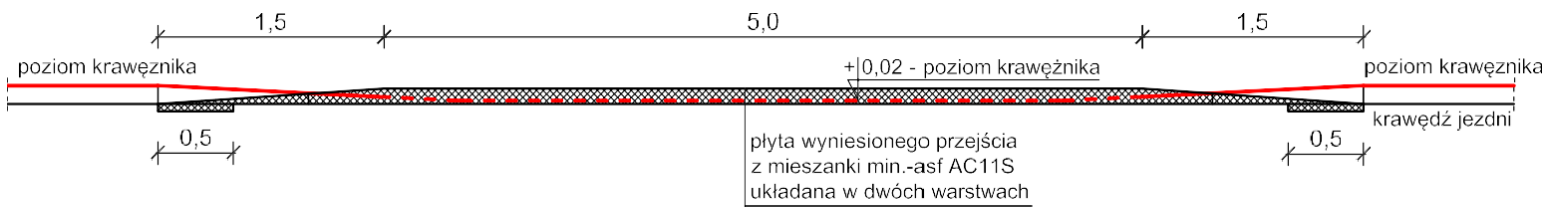
PRZEKRÓJ A-A
