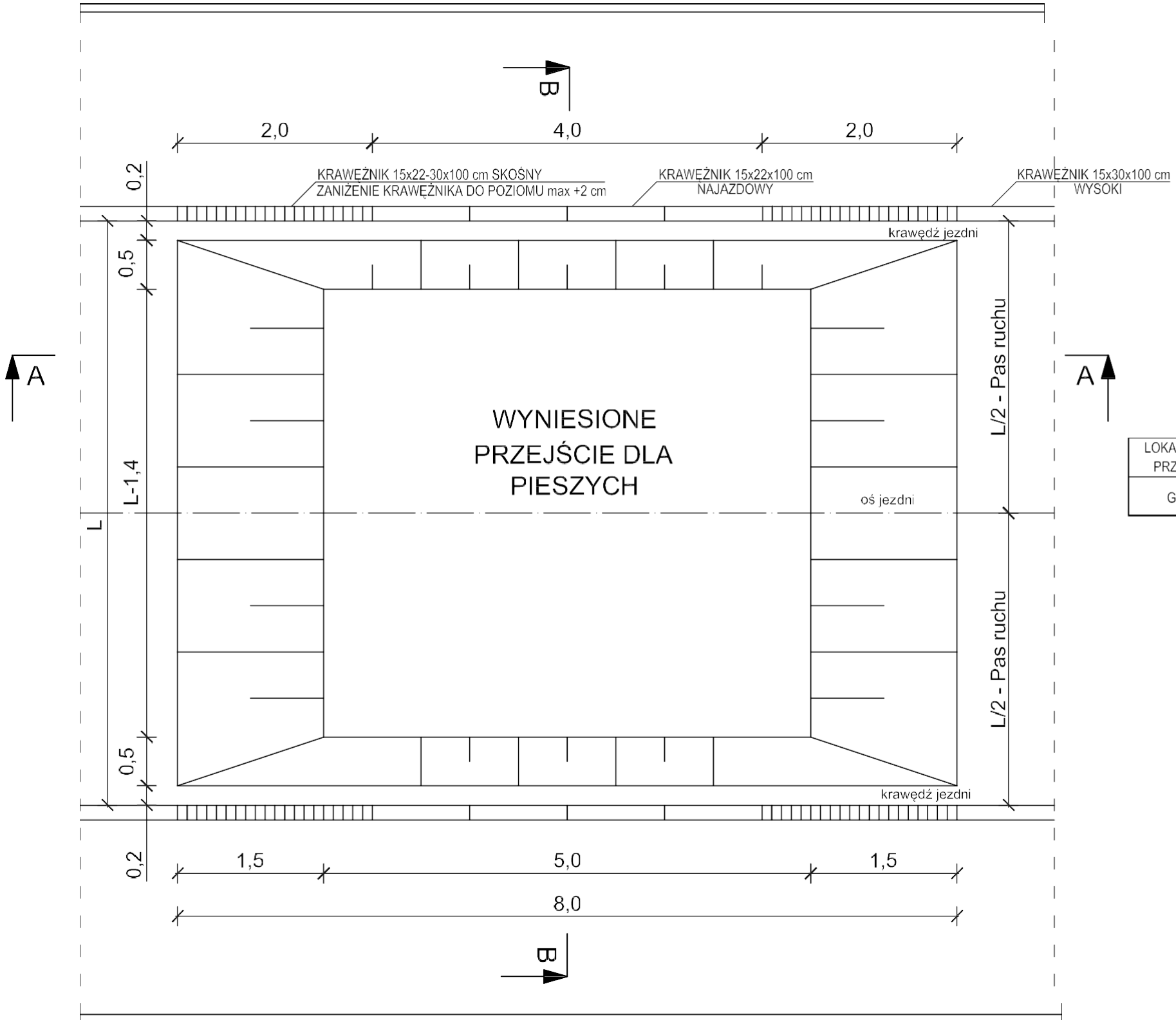
RZUT POZIOMY
