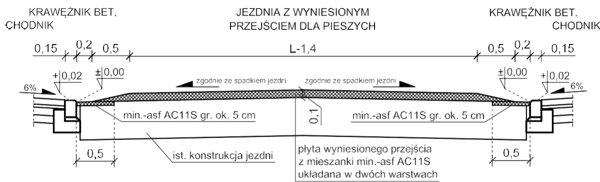
PRZEKRÓJ B-B
