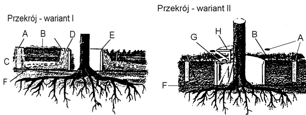
Rys. 5. Studzienka zabezpieczająca pień drzewa przy podwyższeniu terenu powyżej 0,5 m
