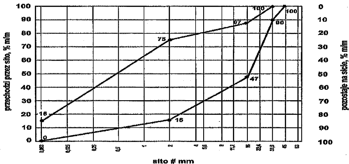
Rys. 1. Krzywe graniczne uziarnienia mieszanki kruszywa niezwiązanego 0/31,5 mm do nawierzchni Istotne cechy środowiskowe
