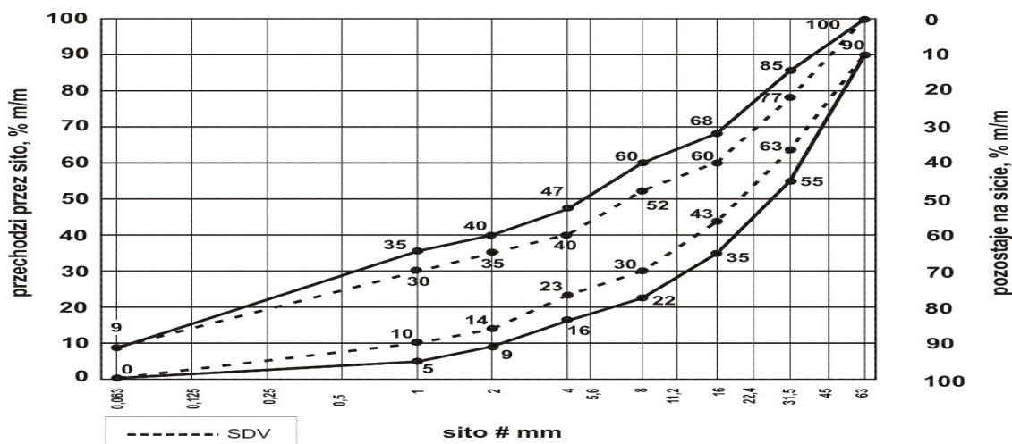
Rys. 4. Uziarnienie mieszanki niezwiązanej 0/63 dla podbudowy zasadniczej
