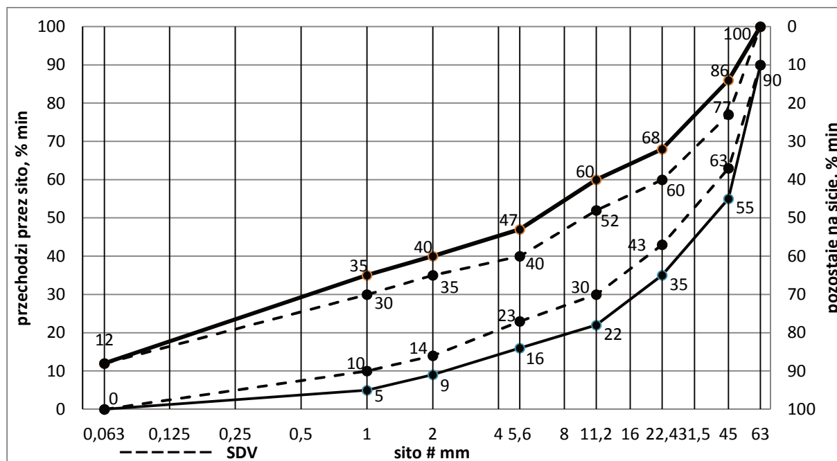
Rysunek 1. Mieszanka niezwiązana 0/63 do warstwy ulepszonego podłoża stabilizowanego georusztem
