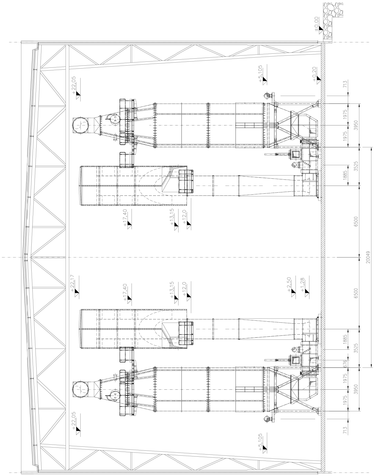
PRZEKROJE "D-D" (SECTION "D-D")
