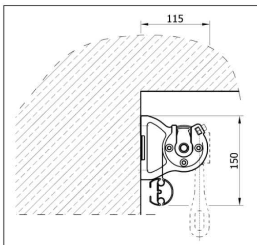
Montaż ścienny - wsporniki standardowe 936XL
