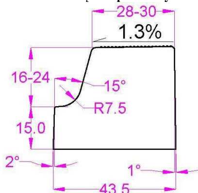
Przekrój poprzeczny krawężników peronowych autobusowych
