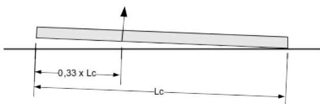
Rys. 2. Schemat pracy żelbetowego pala prefabrykowanego w czasie podnoszenia do kafara
