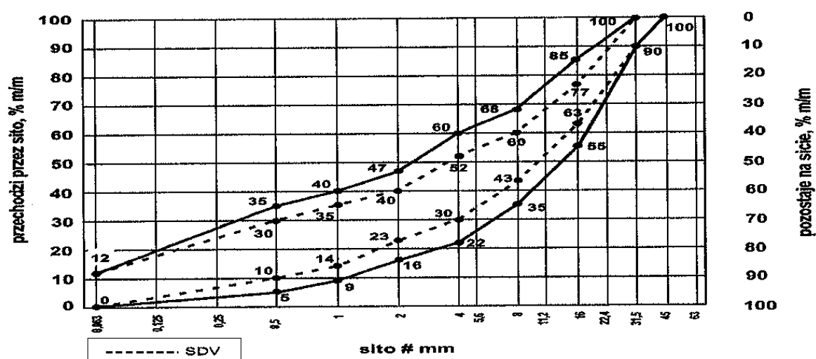
Rys. 3. Krzywe graniczne uziarnienia mieszanki kruszywa niezwiązanego 0/31,5 mm do warstw podbudowy pomocniczej
