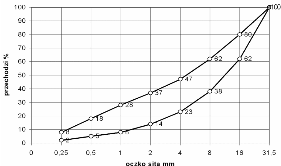
Rysunek 1. Graniczne krzywe uziarnienia kruszywa 0 \div 31,5 mm (dla betonu klasy poniżej C20/25)
