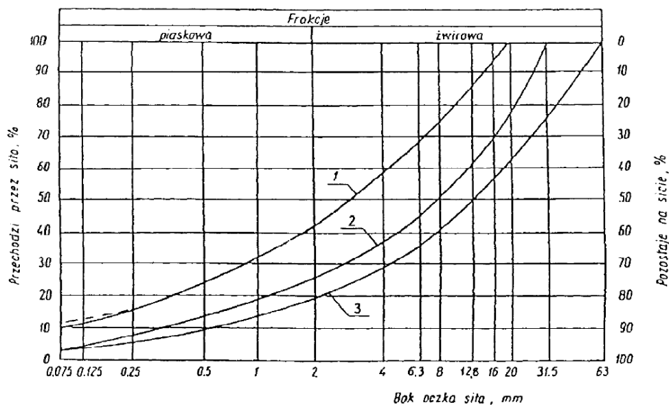
Rysunek 1. Pole dobrego uziarnienia kruszywa przeznaczonych na podbudowy wykonywane metodą stabilizacji mechanicznej: -2 kruszywo na podbudowę zasadniczą (górną warstwę) lub podbudowę jednowarstwową 1-3 kruszywo na podbudowę pomocniczą (dolną warstwę)
