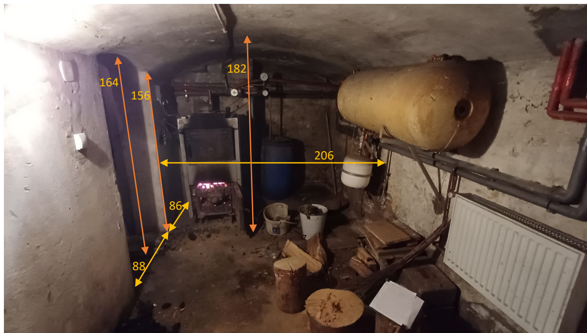
Zdjęcie przedstawia miejsce instalacji kotła wraz z wymiarami.
